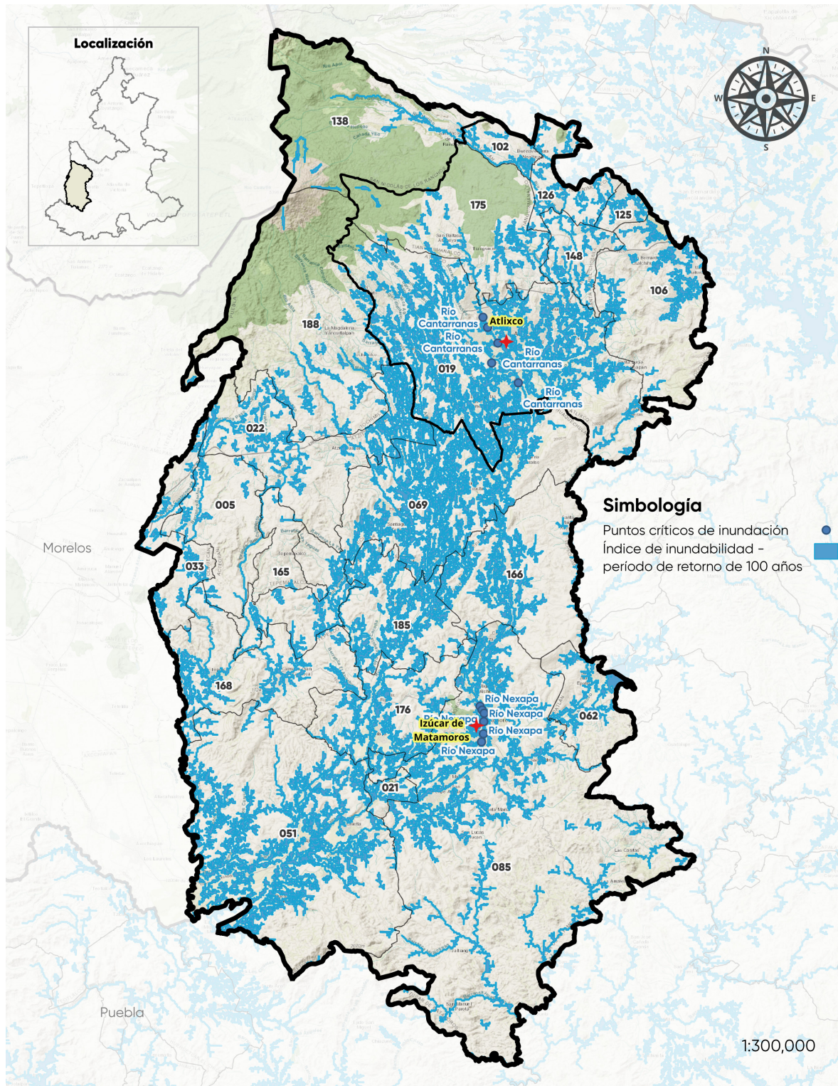
Mapa 6. Riesgo de Inundación
