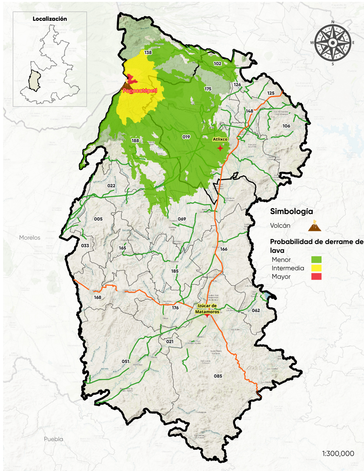
Mapa 8. Riesgos geológicos (peligros volcánicos)
