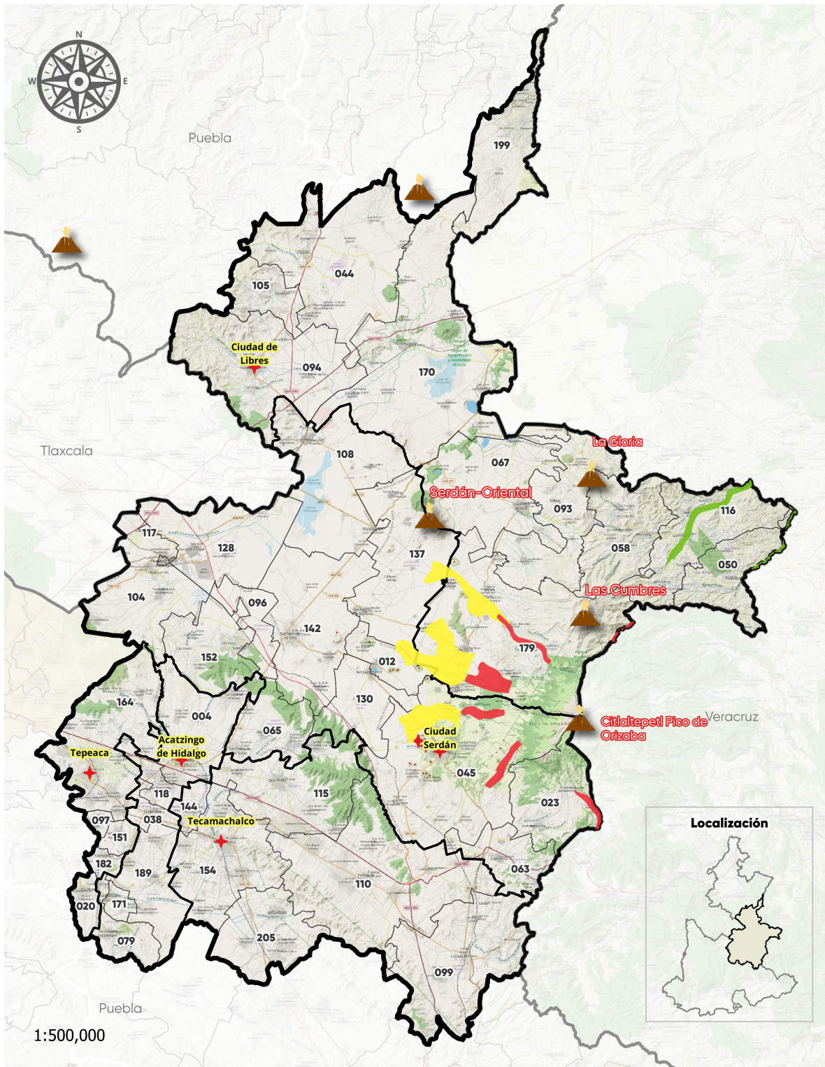
Mapa 9. Riesgos geológicos (peligros volcánicos)
